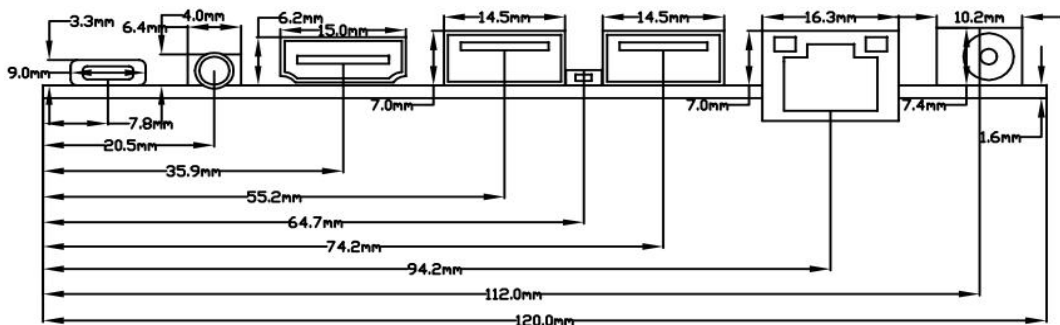
尺寸图
