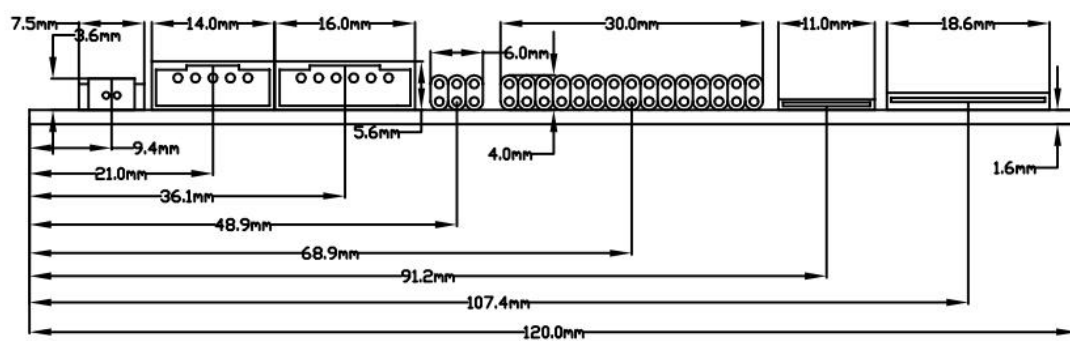
尺寸图
