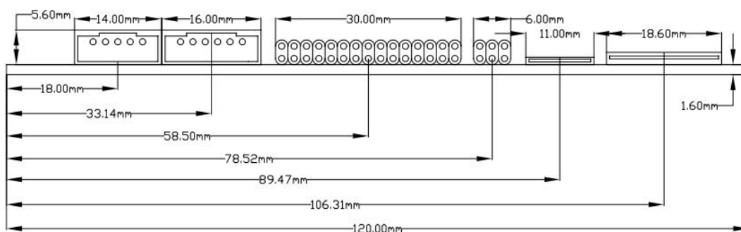
尺寸图
