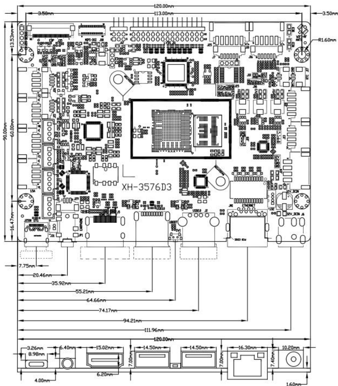
尺寸图
