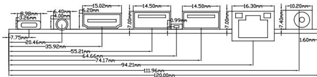
尺寸图
