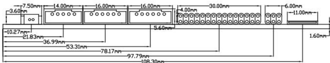
尺寸图
