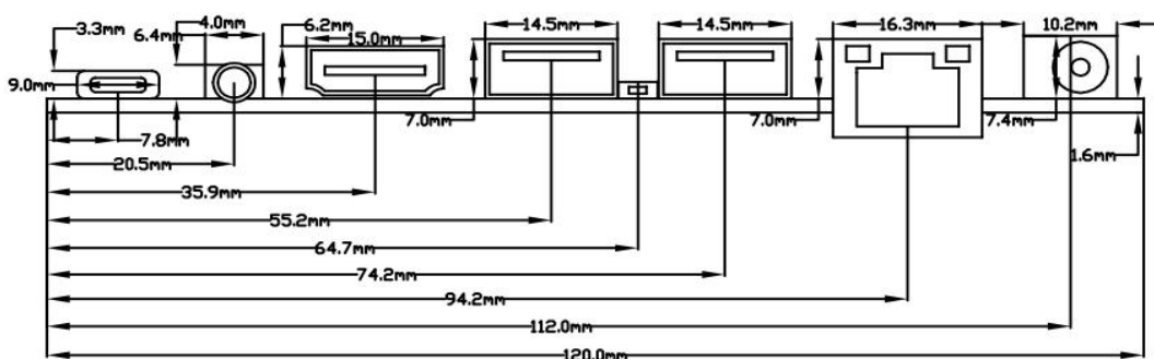
尺寸图
