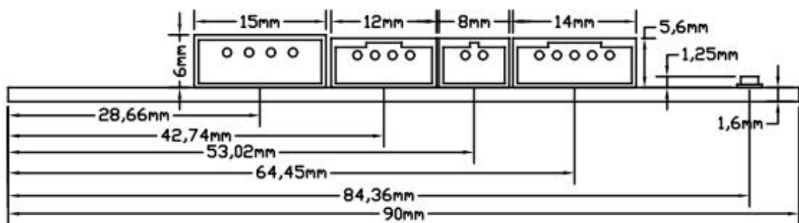
尺寸图
