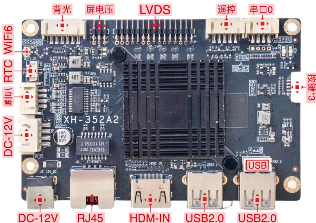
正视图
