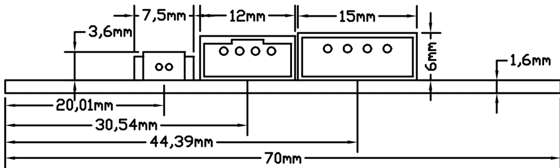
尺寸图
